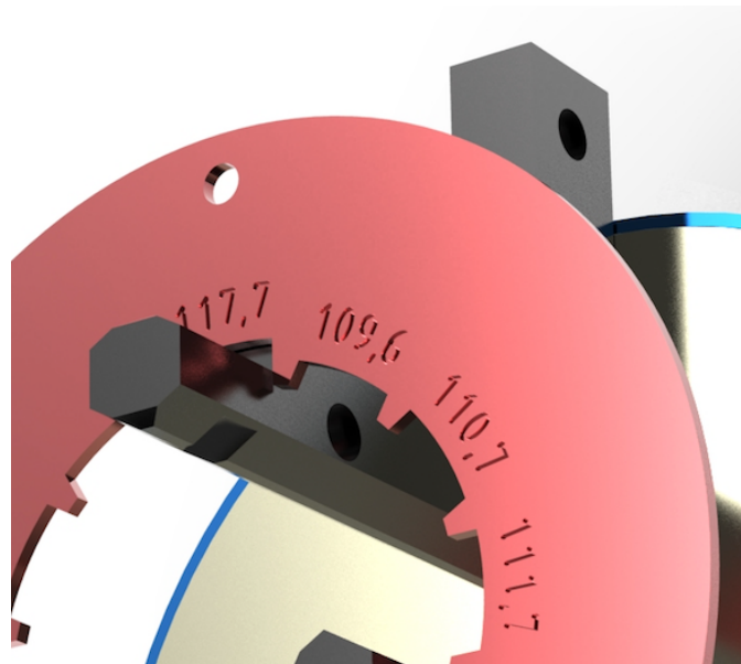
Abbildung zeigt Einrichthilfe für Innenzentrierungen (4-Bereiche). Material: Aluminium / eloxiert
