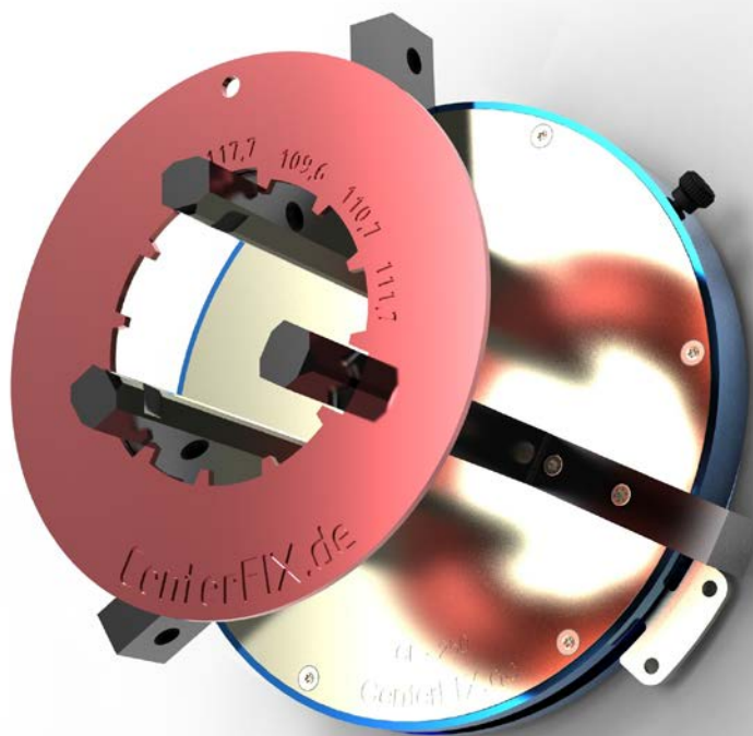
Abbildung zeigt Einrichthilfe für Innenzentrierungen (4-Bereiche). Material: Aluminium / eloxiert
